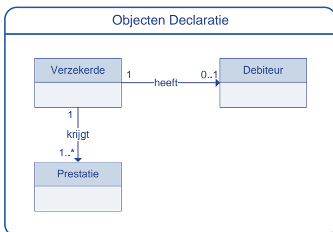
Figuur 4-1 Objectmodel Declaratie ZZP en extramurale parameters forensische zorg
