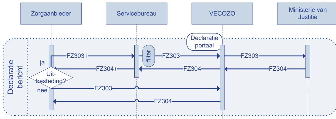
Figuur 3-1 EI-declaratiestromenmodel FZ303-FZ304
