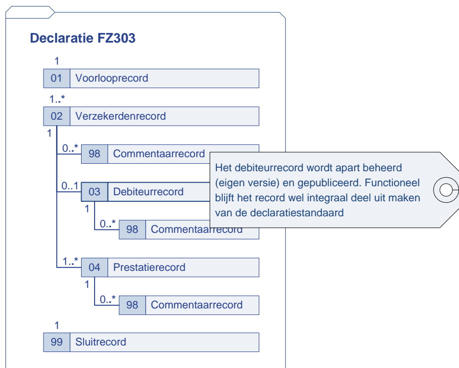
Figuur 5-1 Logische bestandstructuur FZ303
