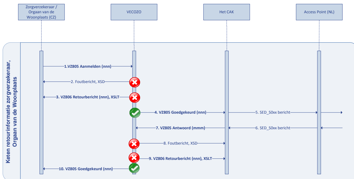
Figuur 6-1 Keten retourinformatie zorgverzekeraar of orgaan van de woonplaats (CZ)
