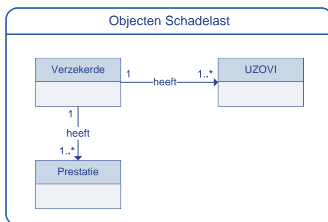
Figuur 4-1 Objectmodel Schadelast Verloskundige hulp
