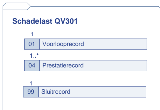
Figuur 5-1 Logische bestandstructuur Aanleverspecificaties schadelastinformatie Verloskundige hulp
