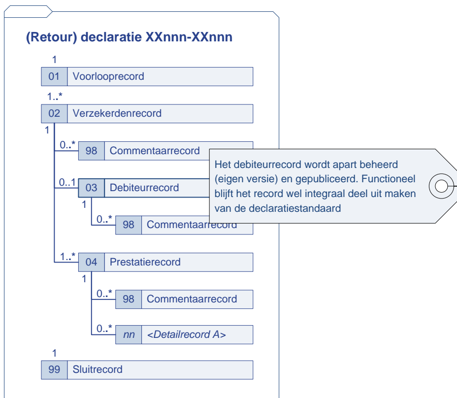
Figuur 6-3 Logische structuur EI-retourinformatiebericht bij deels afgekeurd EI-declaratiebericht
