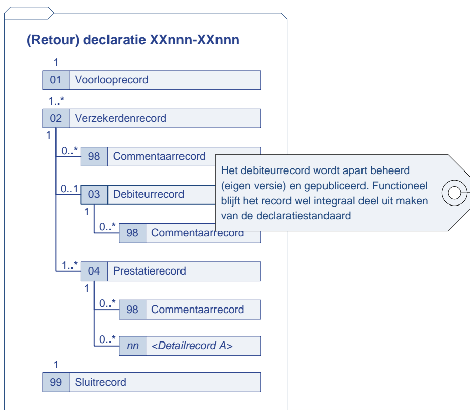
Figuur 5-1 Logische bestandstructuur KZ301v3.2
